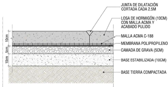
DETALLE CONSTRUCTIVO RADIER DE HORMIGÓN
